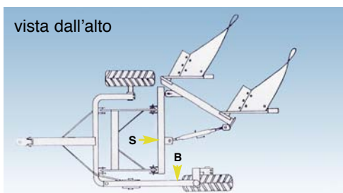
Carrello completo di aratro bivomere con supporto "S" e braccio "B" per ruota pivotante Trailer and plough with 2 shares and "S" support and "B" arm for pivot wheel.
